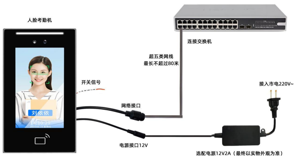
D76D78 考勤模式下接线图
