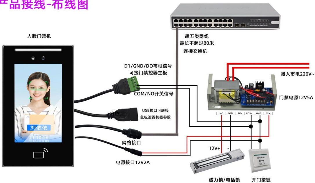
D76D78 门禁模式下接线图
